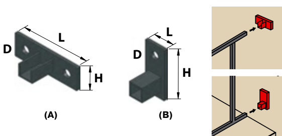
Platine à visser pour poteau balcon (x2)
